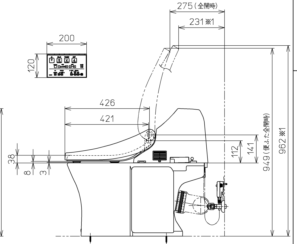
床給水仕様の場合
