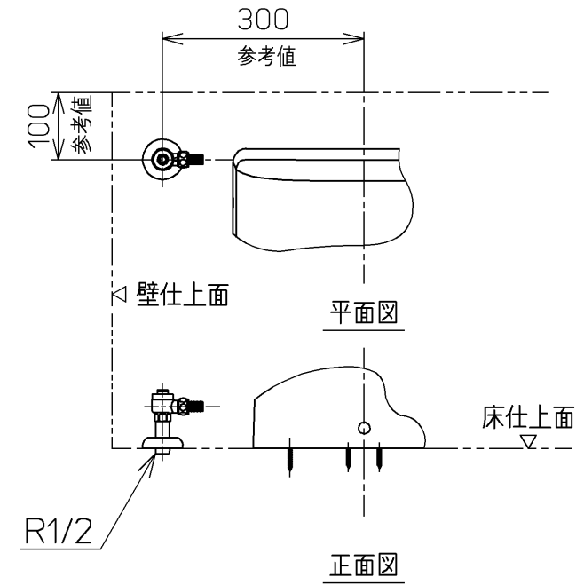
床給水仕様の場合
