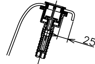
断面B-B(1:5)
