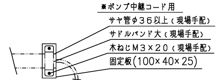
断面B-B(1:5)
