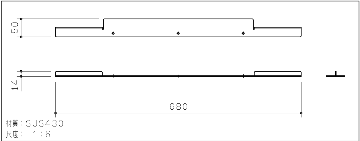
底板支持材
