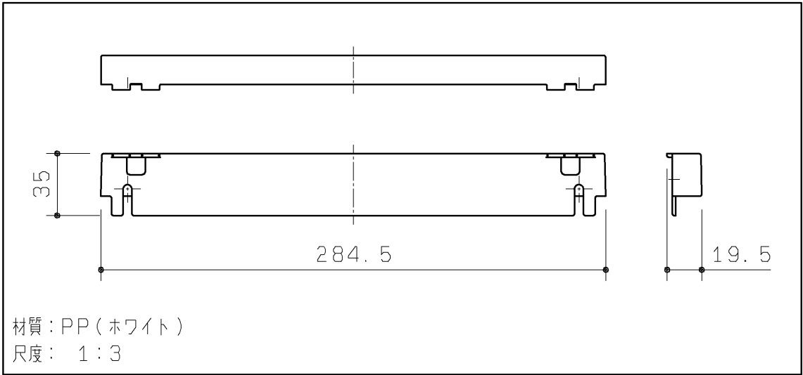
棚板キップ
