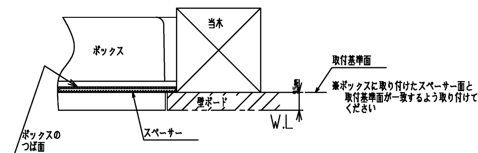
(B) 壁厚みが9.5mmの場合：ボックスのつば面にスペーサーを取り付けてください
