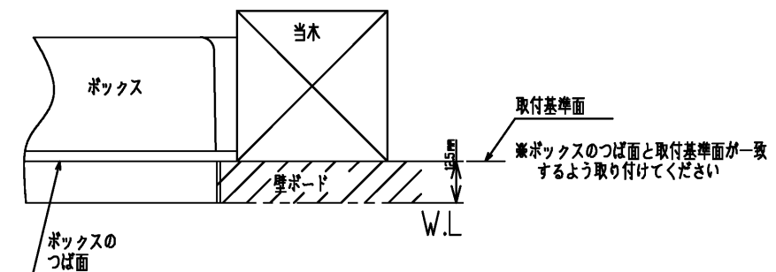
(A) 壁厚みが12.5mmの場合：スペーサーは不要です
