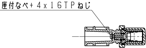
A-A断面 (S=1:3)
