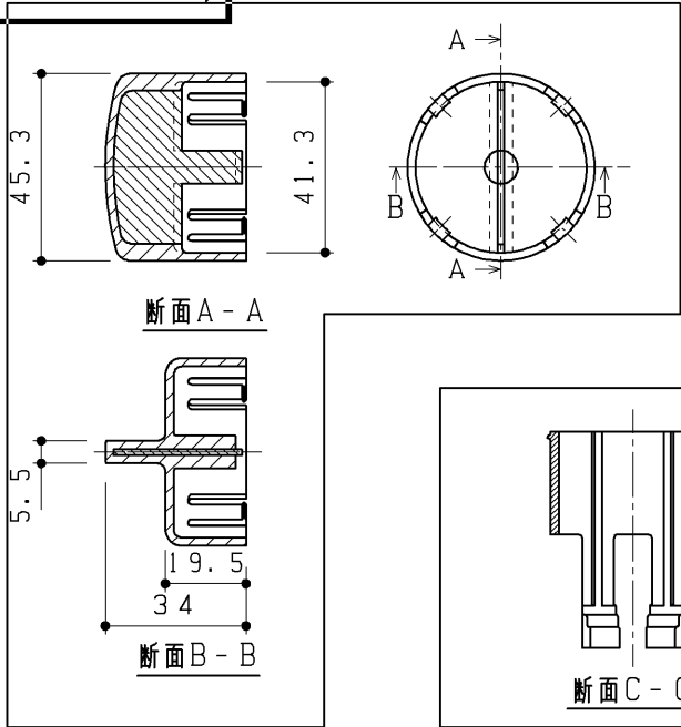
止水栓ハンドル
