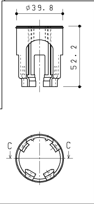
止水栓ハンドル取付材
