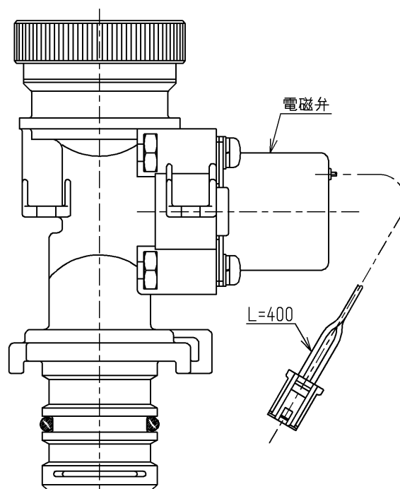
駆動部 (2個)
