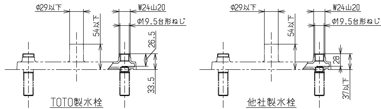
取付可能な水栓の主要寸法
