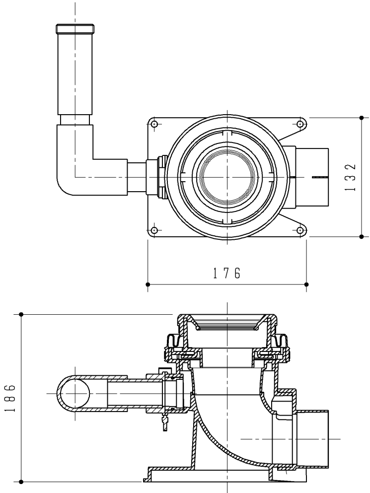
手洗排水管（間口調整用）
