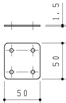
(S=1:3) 材質: SUS304
