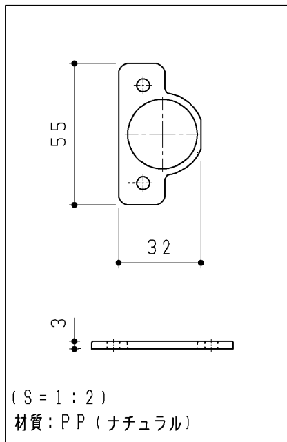
丁番用スペーサー (2ヶ)
