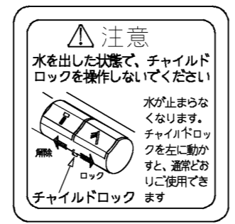
※2 注意ラベル詳細(1:1)
