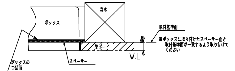
壁厚み別ボックス取り付け位置詳細図
