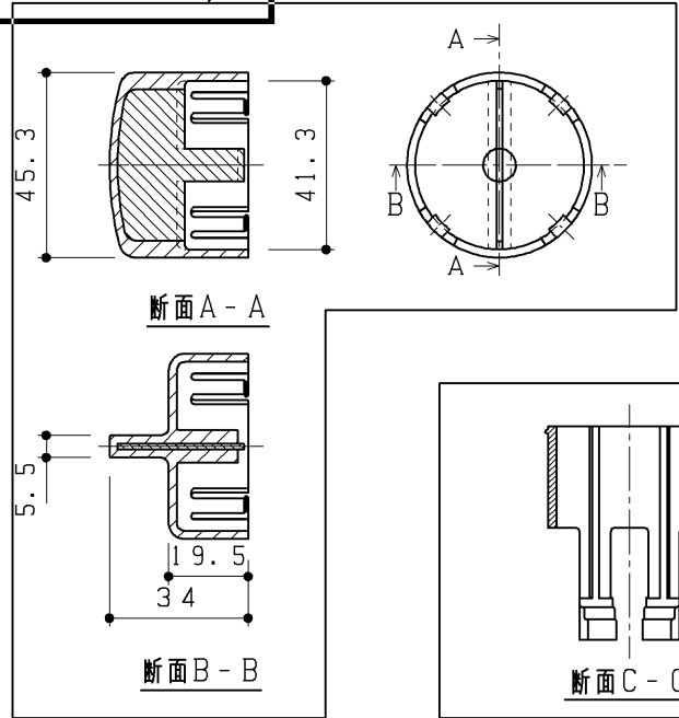
防露カバー(止水栓用)
