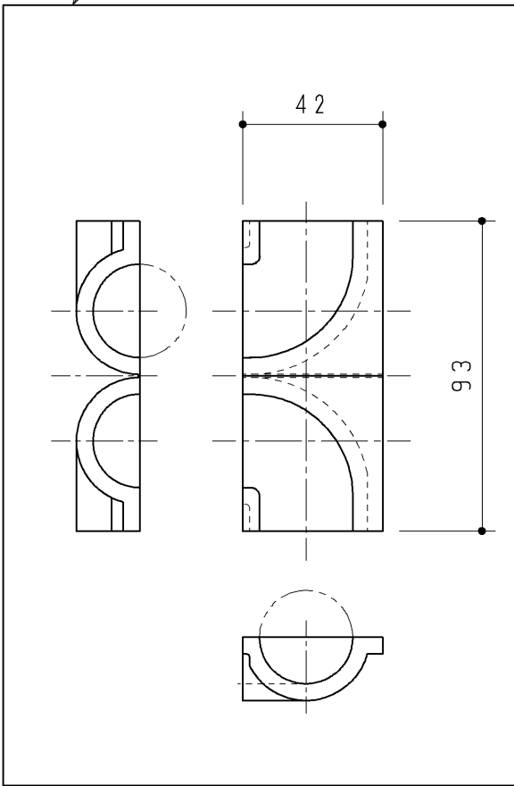
防露カバー(オスメスエルボ用)
