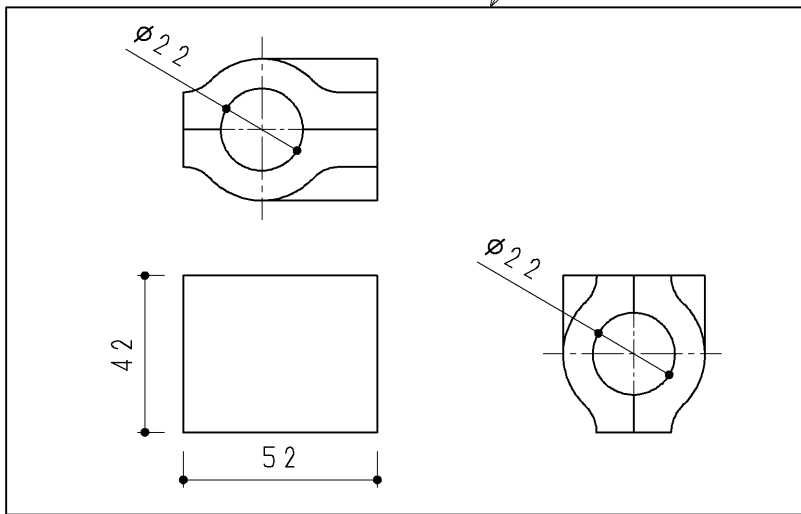
防露カバー(分岐金具部)
