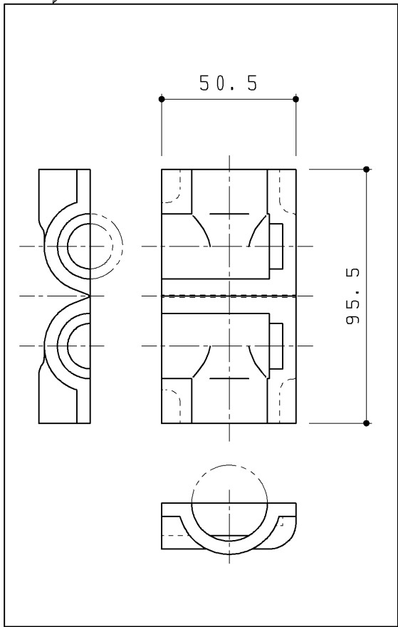
防露カバー(エルボ部、WL用)
