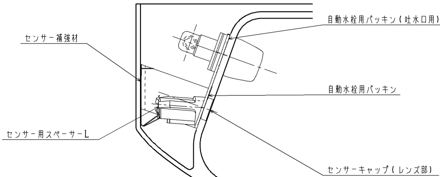
A部断面詳細図（S=1：2）
