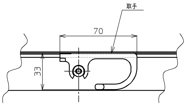
B-B' 断面拡大図(S=1/2)
