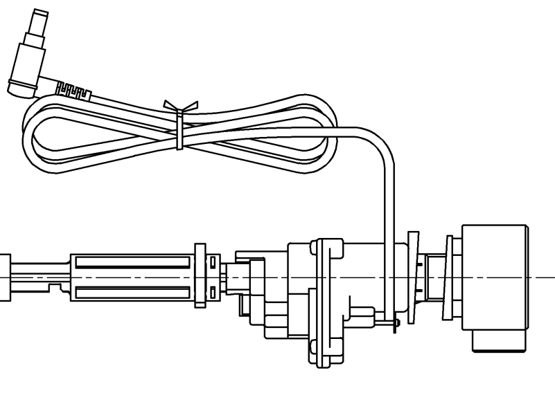
レスティカ・CSR (CS680系)・NEW CS (C770系) / 寒冷地仕様の場合
