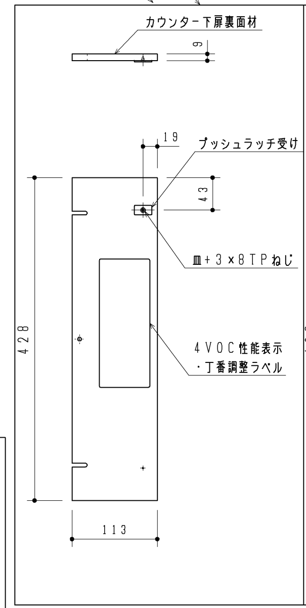
カウンター下扉表面材
