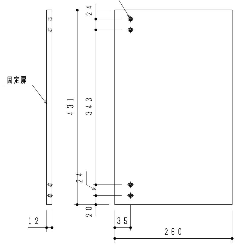
側板目地材L
