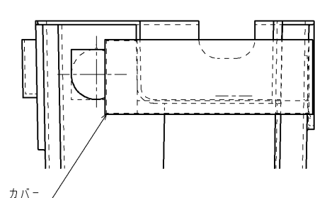
C 視図
