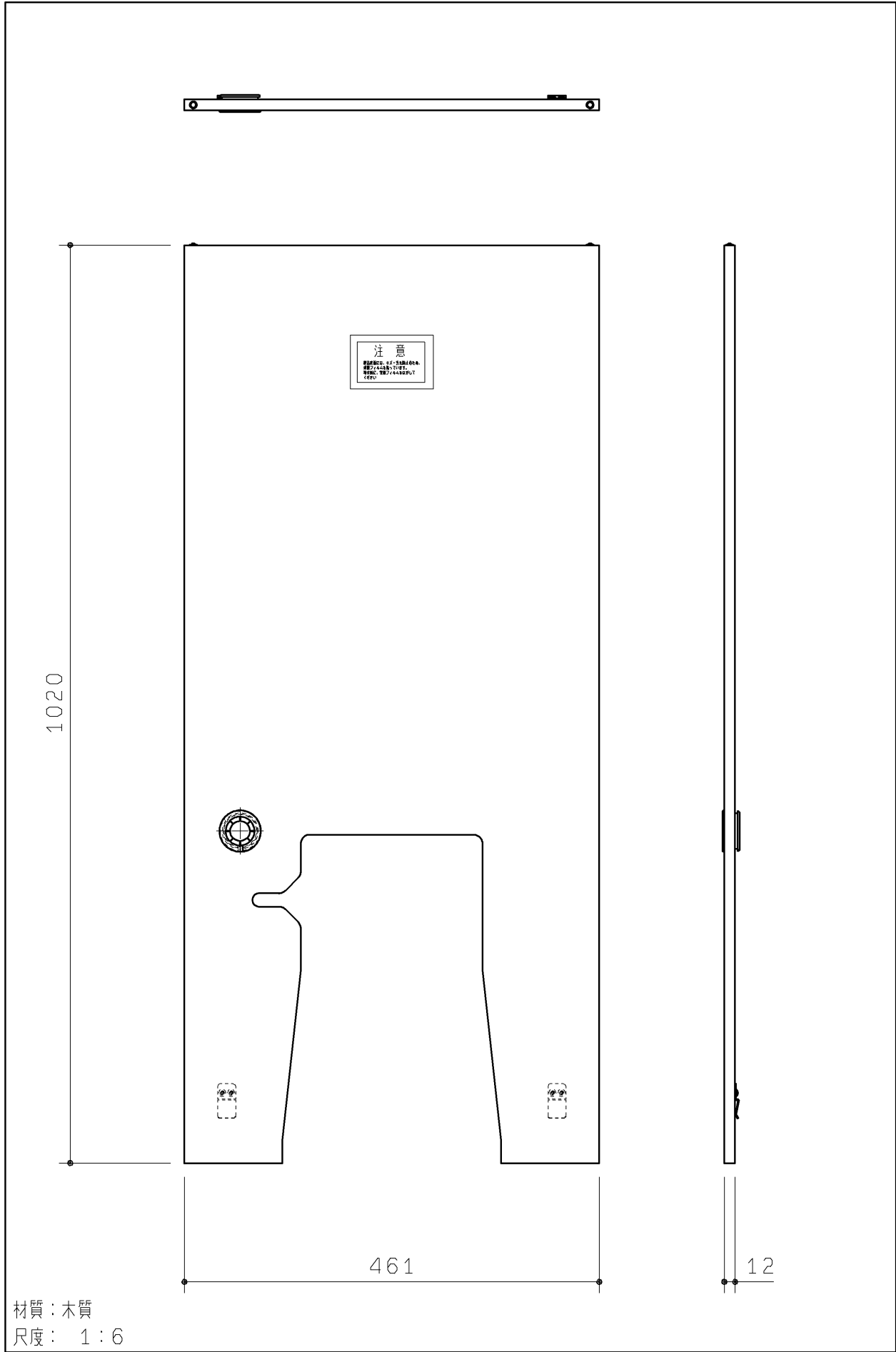
前板セット
