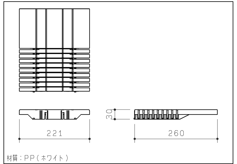
棚板(2ヶ)
