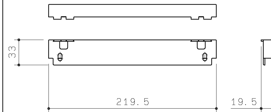
底板支持材
