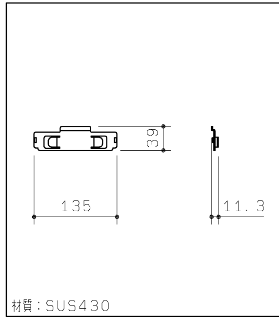
棚板支持材セット(2ヶ)
