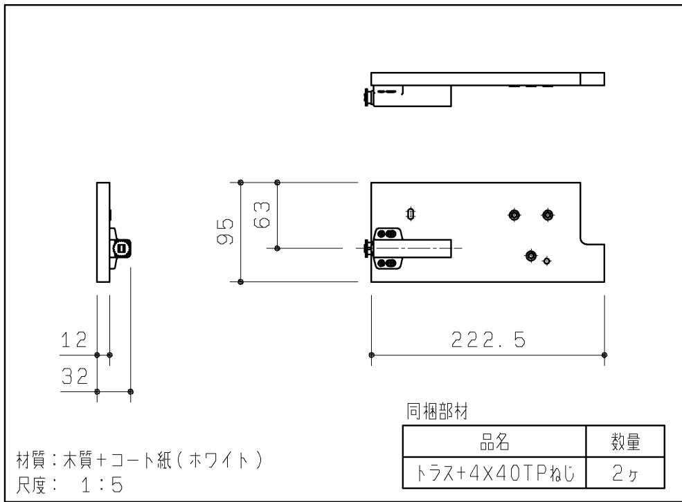
壁側板セット左
