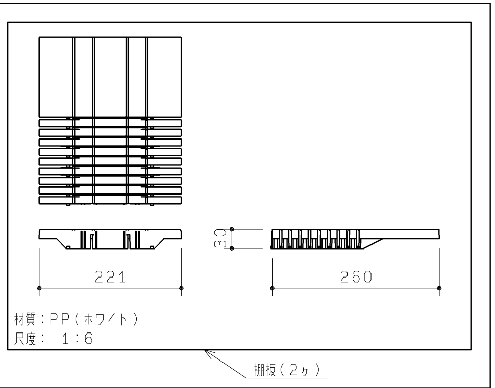
棚板セット(2ヶ)
