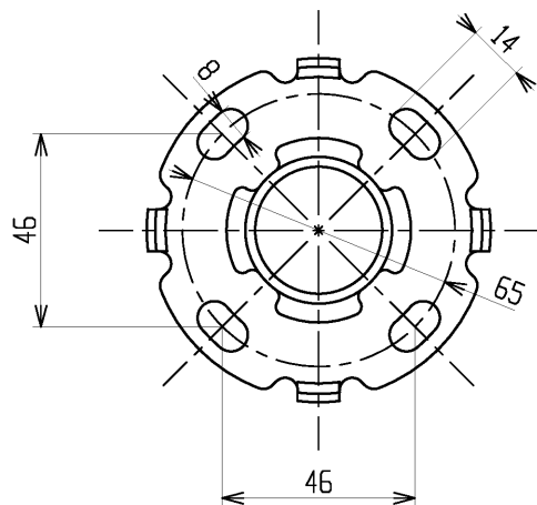
取付座詳細(1:2)
