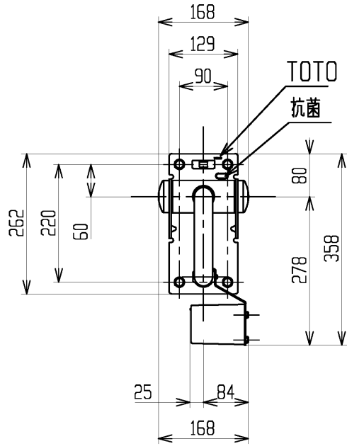
右勝手の場合 (便器に向かって右側に手すりを設置する場合)
