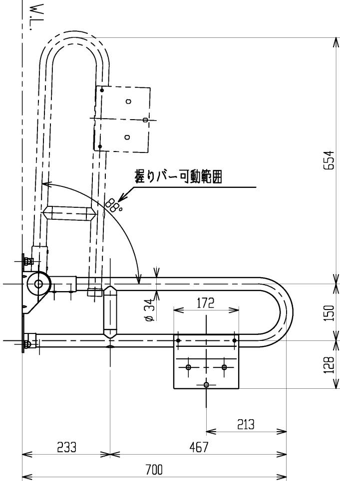
左勝手の場合 (便器に向かって左側に手すりを設置する場合)
