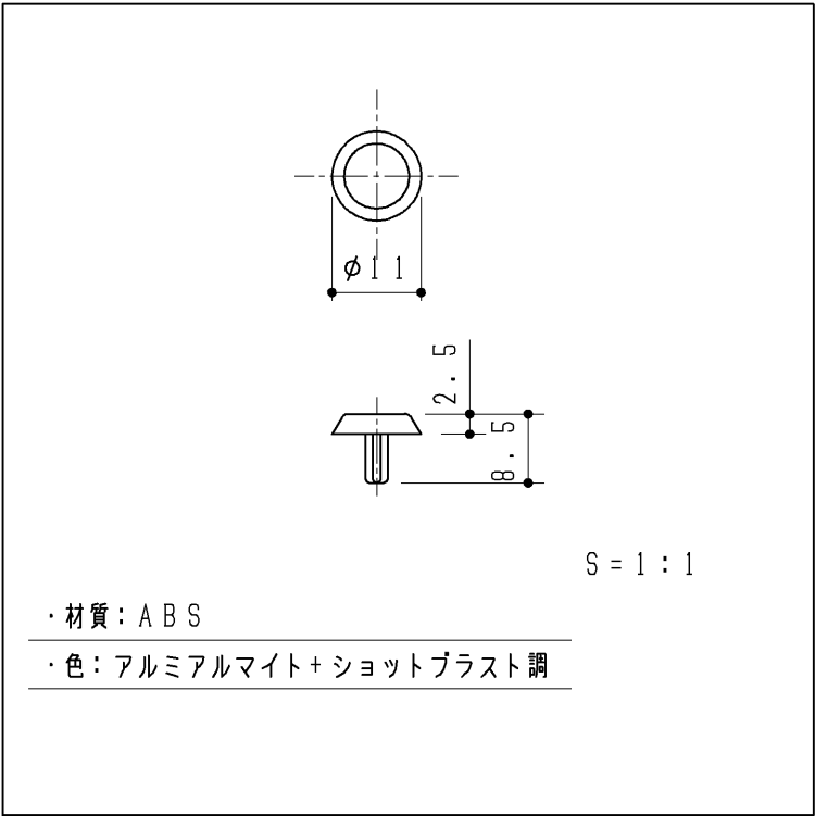
化粧ビス用キャップ 2ヶ
