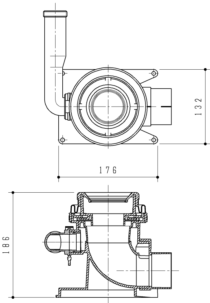
手洗排水管（間口調整用）
