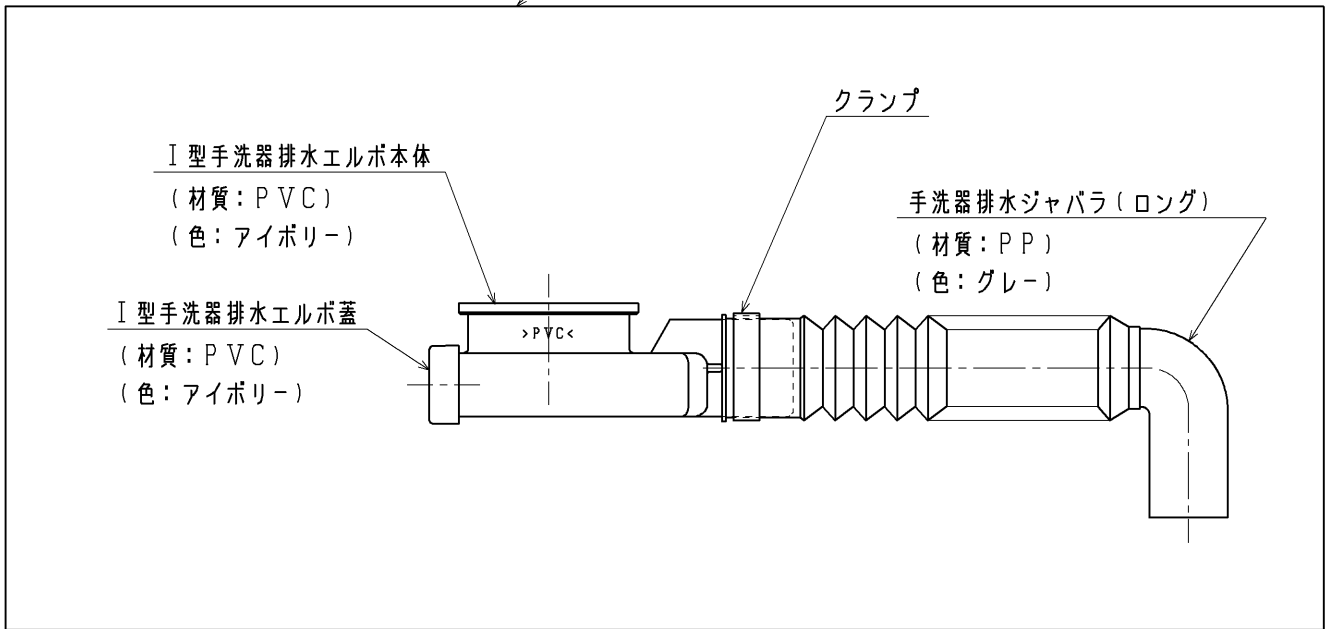
I 型手洗排水エルボセット
