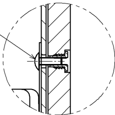
A部詳細 (S=1:2)
