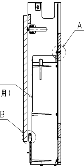
室内暖房ユニット固定詳細
