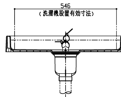
断面B-B
