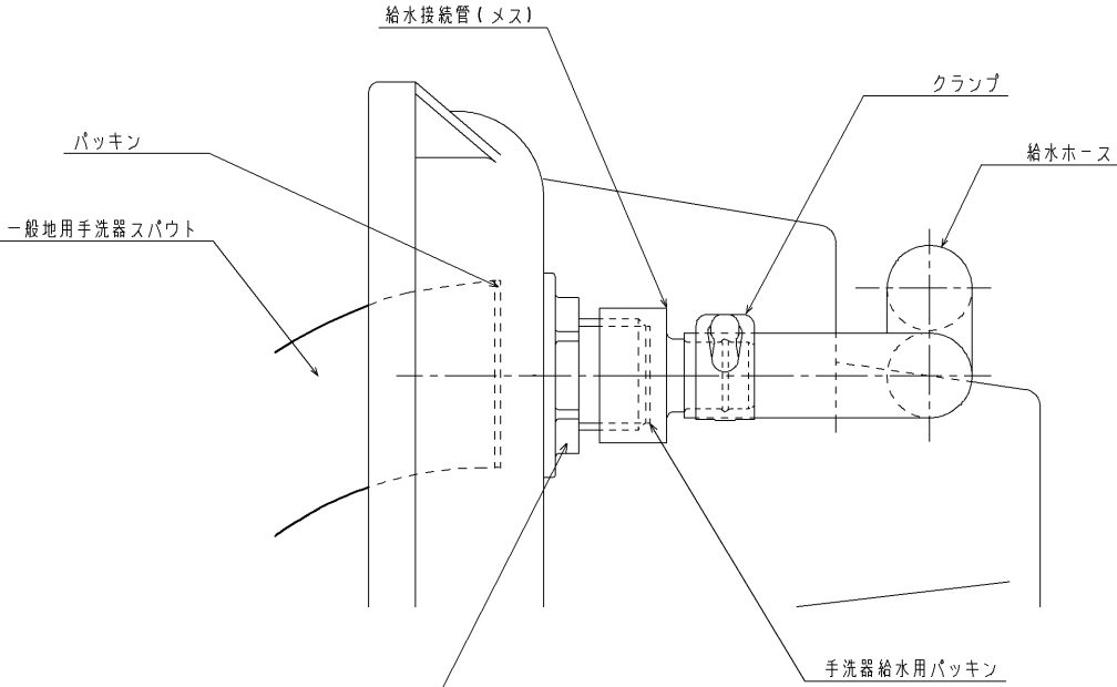
D部詳細図(S=1:1)
