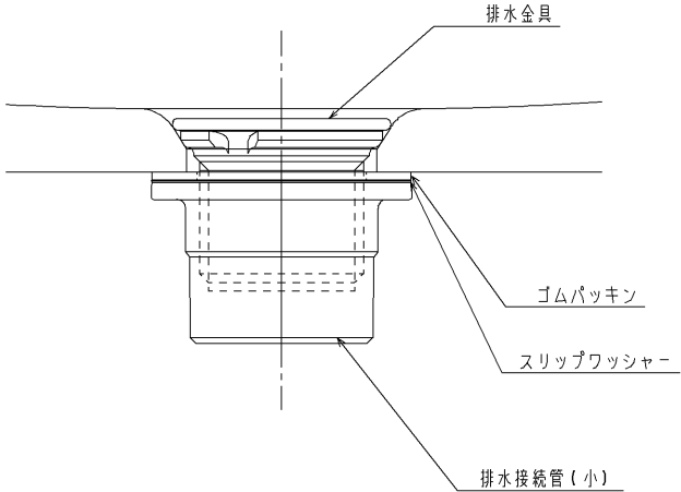
B部詳細図(S=1:1)
