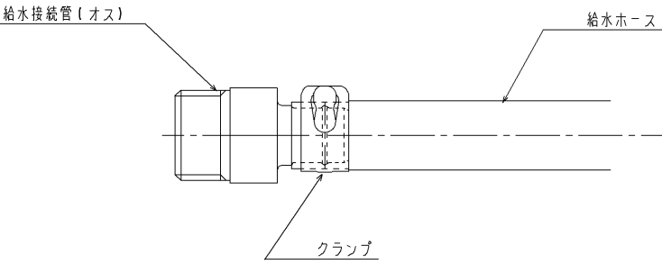
C部詳細図(S=1:1)
