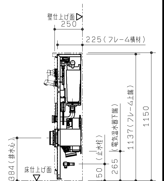
R 視図
