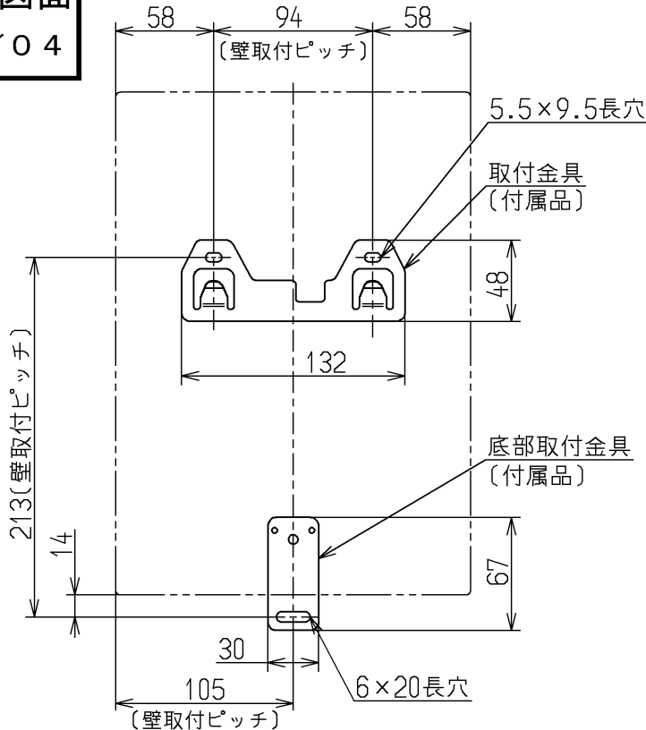
■取付金具詳細図
