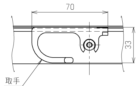
B-B断面詳細図 (1:2)
