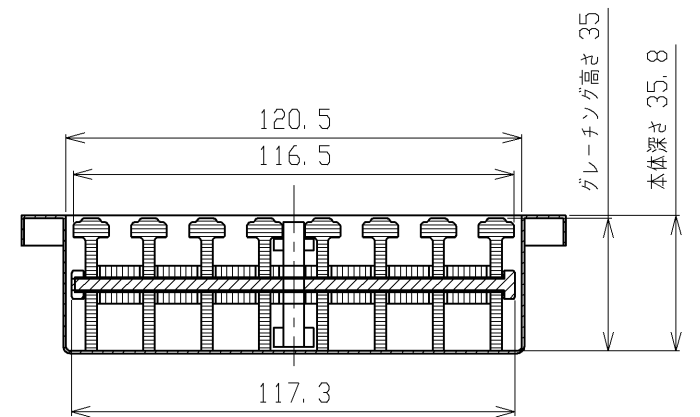
A-A断面詳細図 (1:2)
