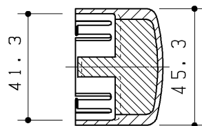
断面B-B
