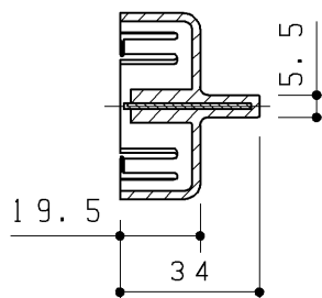
断面A-A
