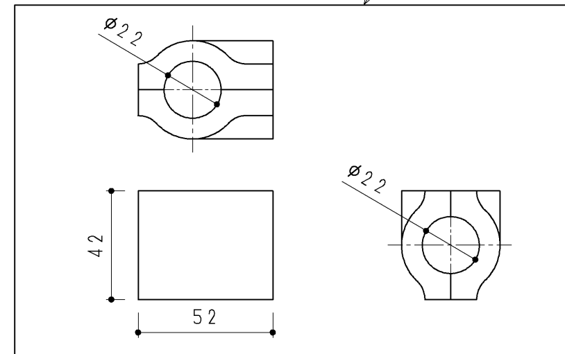
防露カバー(分岐金具部)
