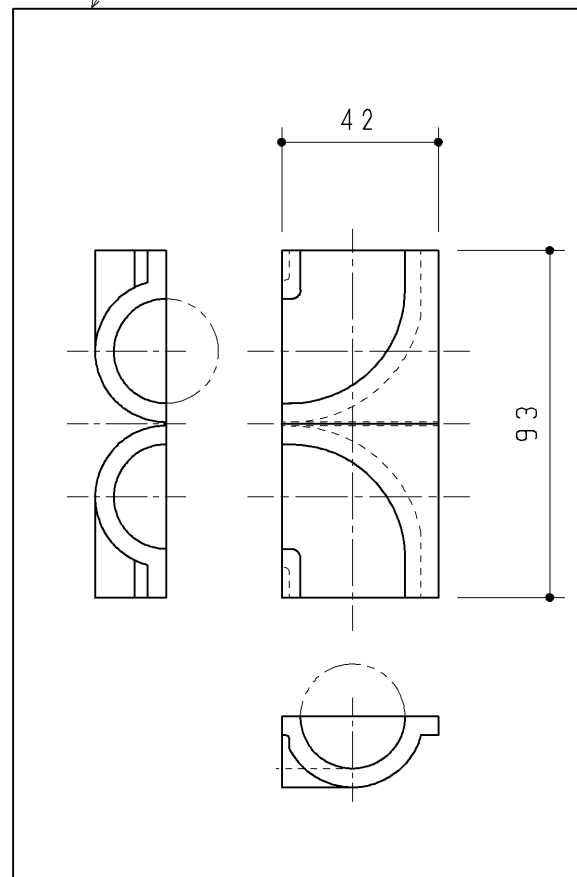
防露カバー(オスメスエルボ用)
