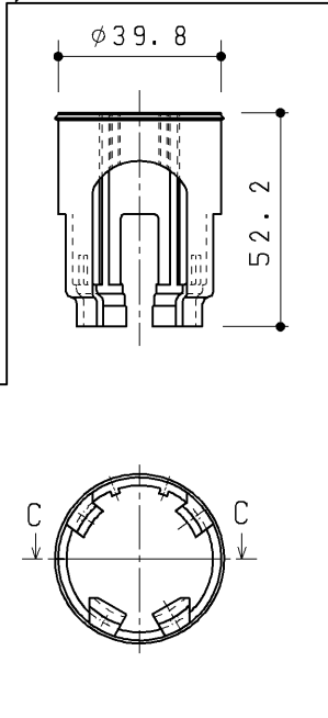
防露カバー(エルボ部、WL用)
