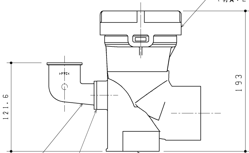
手洗排水管 （材質：PVC）
