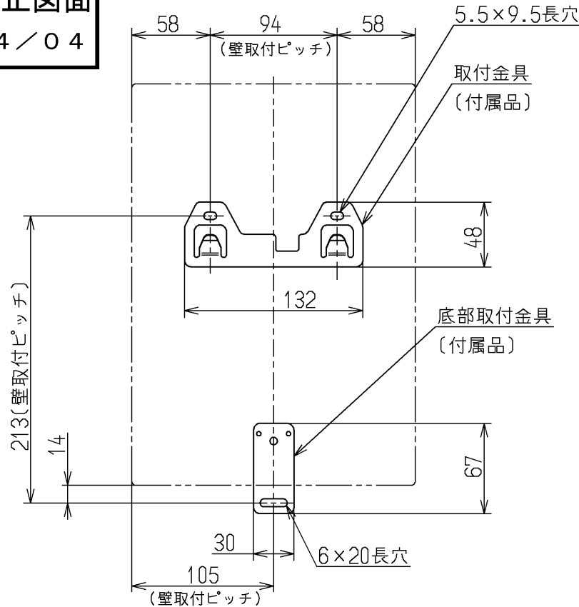
■取付金具詳細図
