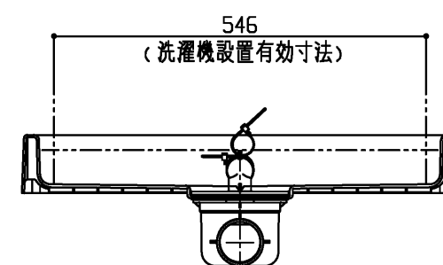
断面B-B
