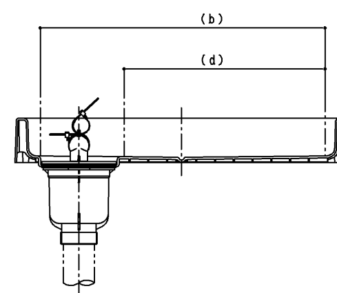
断面B-B
