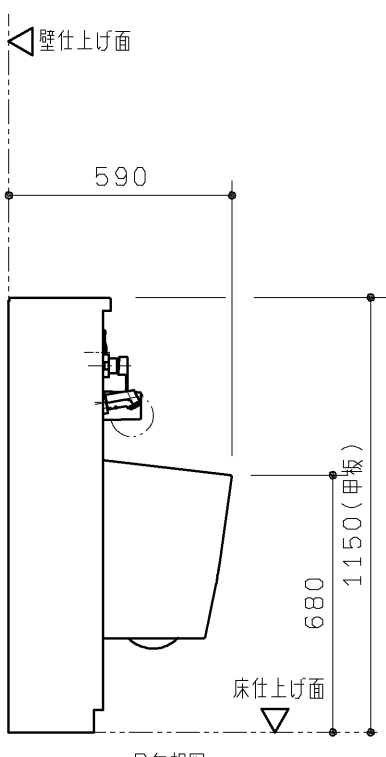
B矢視図
