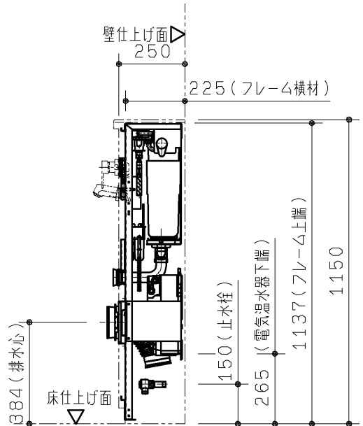
R 視図
