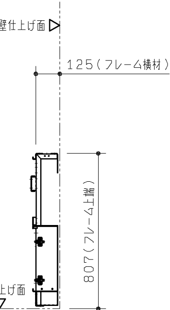
Q 視図
