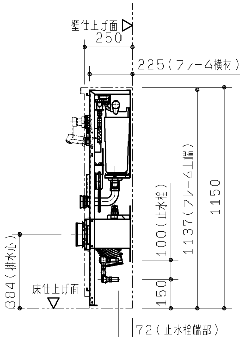
R 視図
