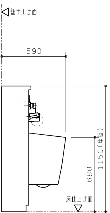
B矢視図
