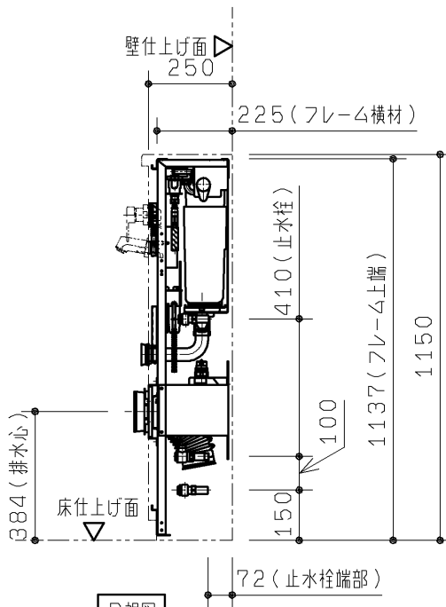
R 視図
