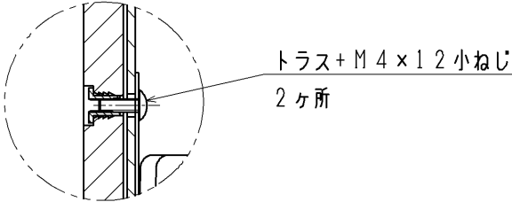
A部詳細 (S=1:2)
