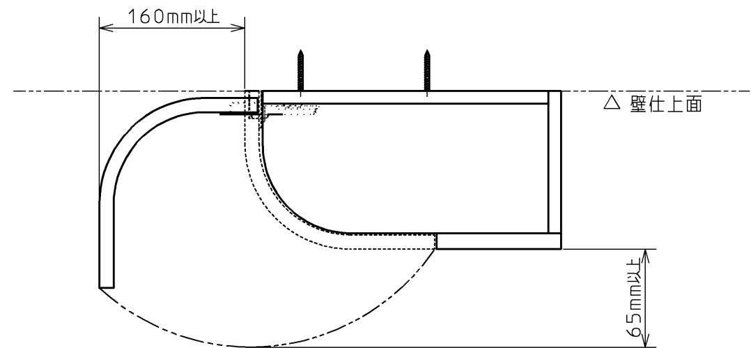
開口状態図
