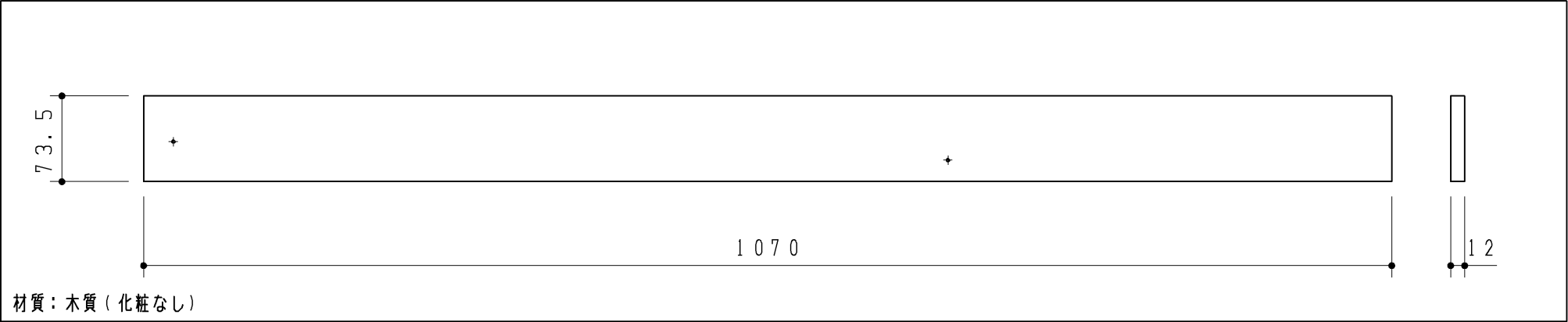
下段補強桎
