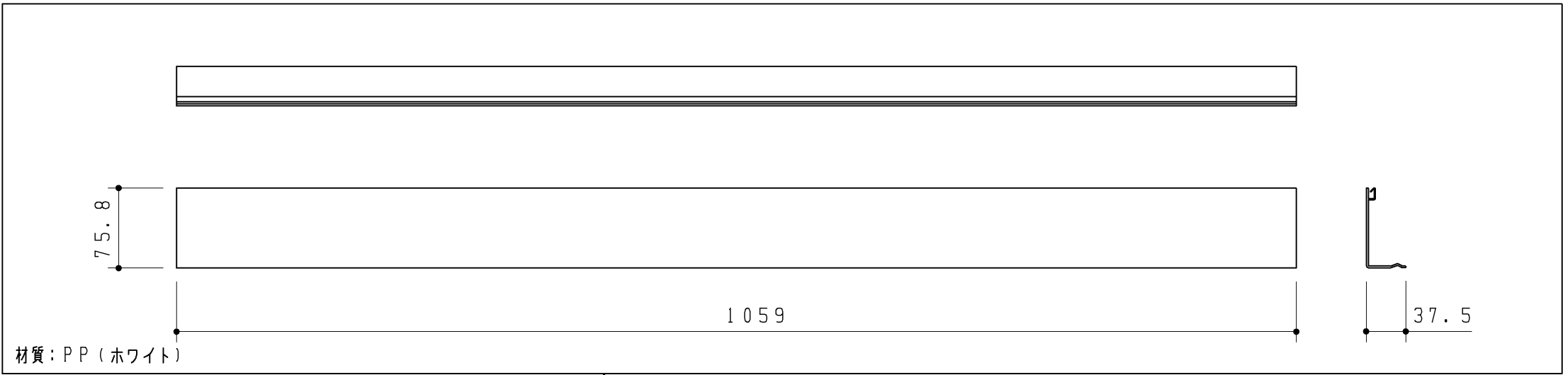
配管カバー
