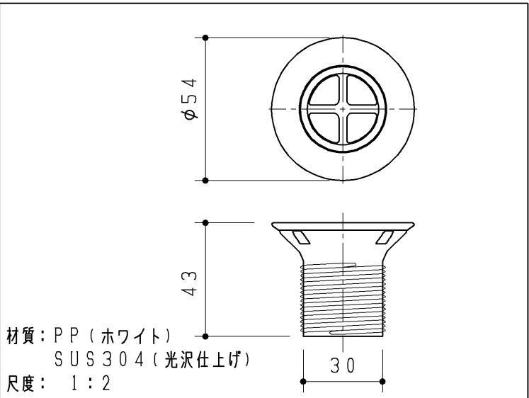
排水金具
