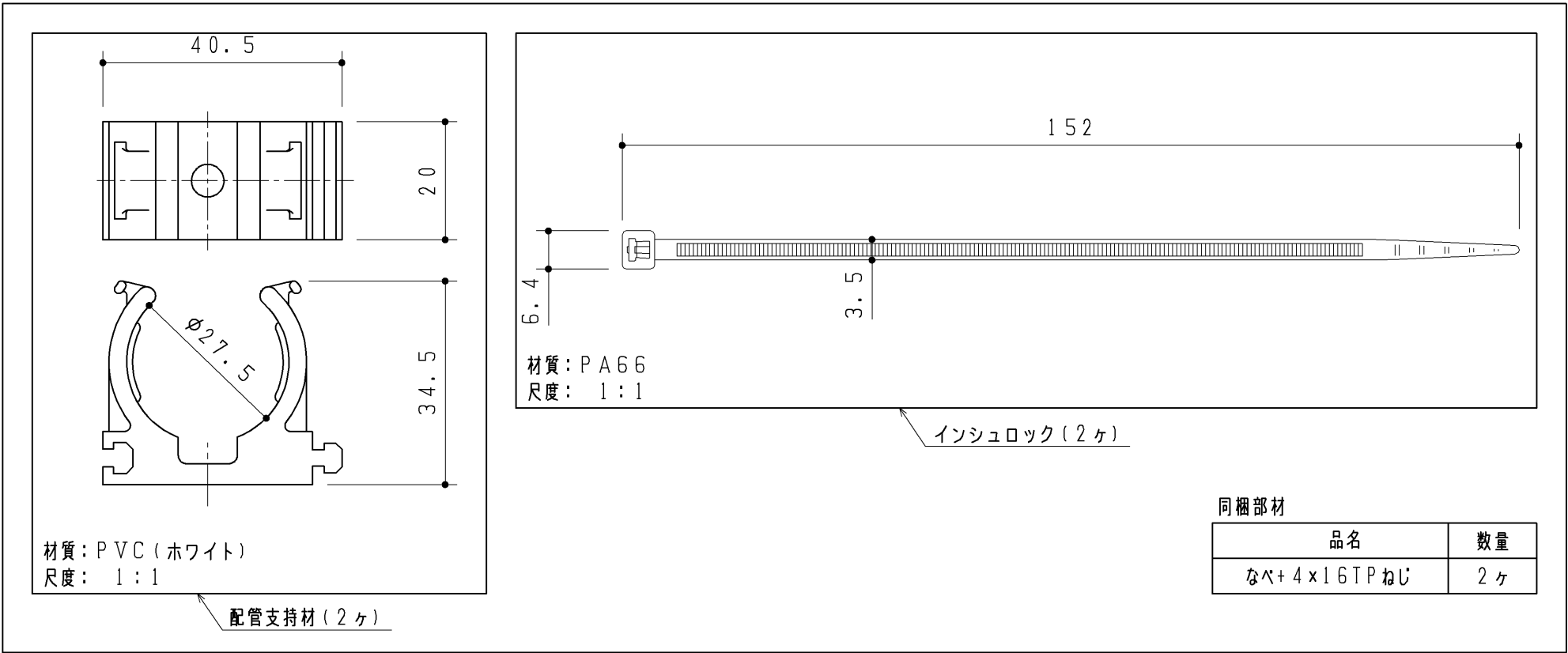
配管支持材セット
