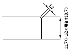
A部（面取り部）拡大図
