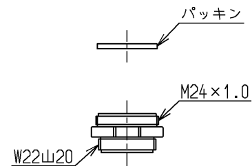
吐水口ねじ変換用 アダプター(1:2)
