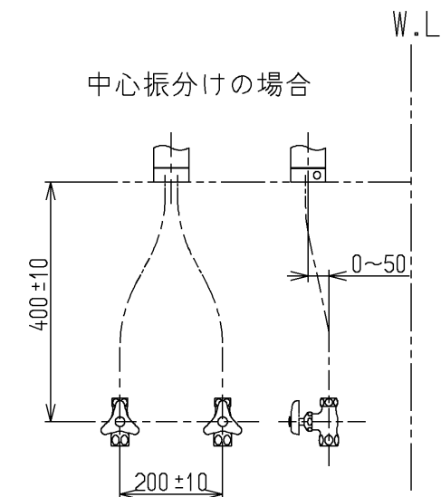
止水栓推奨取付位置
