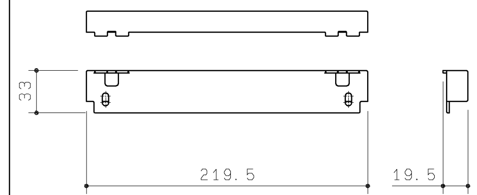
底板支持材
