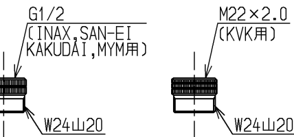
取替え接続用アダプタ
