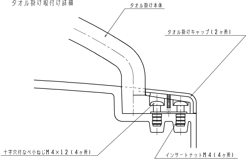
タオル掛け取付け詳細
